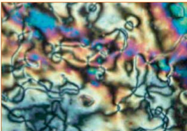
(b) 液体から液晶が出てくるところ
