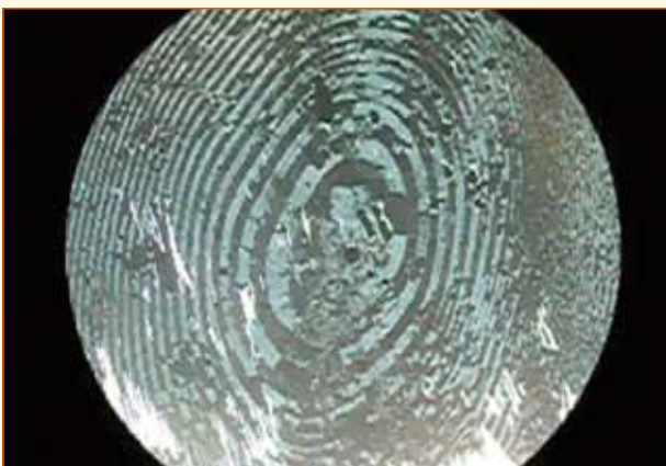
図2 偏光顕微鏡で観察した液晶の模様
