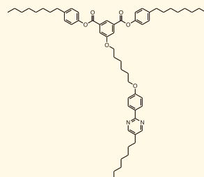
図3 アモルファスブルー相IIIを用いた表示素子とその鍵化合物
