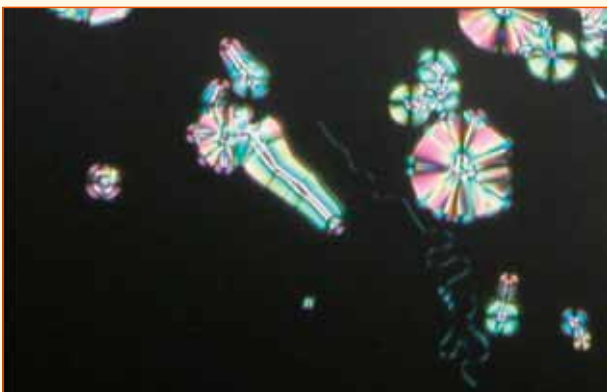
(b) 液体から液晶が出てくるところ
