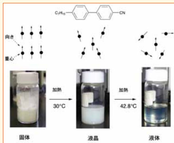
図1 液晶の外観と秩序
