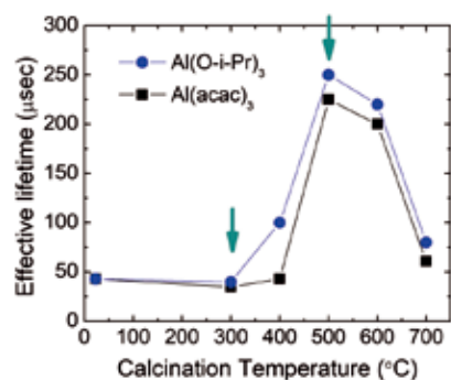
図1：アルミナパッシベーション膜のキャリア寿命—試料焼成温度依存性
